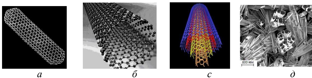
Рисунок 1.25 – Схематическое изображение углеродной нанотрубки (а) и расположение атомов на ее поверхности (б); многослойная нанотрубка (с); «колонии» углеродных нанотрубок (д)
