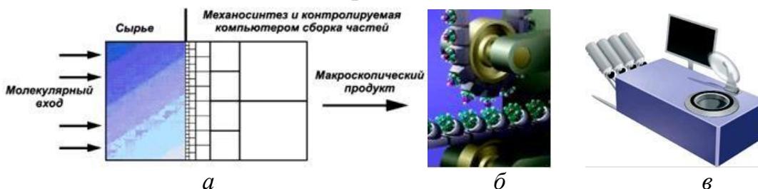
Рисунок 1.6 – Атомно-молекулярная сборка изделий с помощью ассемблера: а – схема процесса генеративной сборки продукции на наноуровне; б – предполагаемая производственная линия наносборки; в – возможный вид нанофабрики
