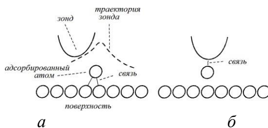
Рисунок 1.7 – Иллюстрация траектории острия зонда СТМ над адсорбированным на поверхности материала атомом: а – режим изображения (острие зонда не контактирует с поверхностью, но располагается достаточно близко для получения изображения);
